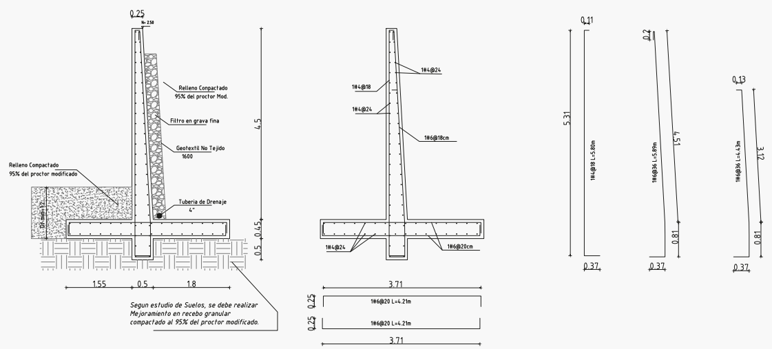
DETALLE DE MURO TIPO 1 (M-T1) desde K0+008 hasta K0+0.28
